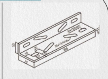
2MC062
