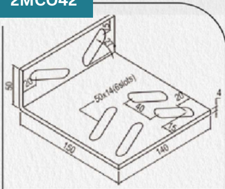
2MCO42
